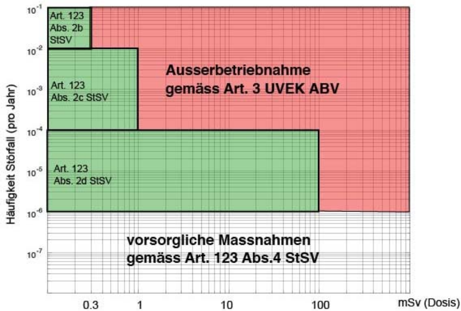
Abbildung 1: Gesetzliche Vorgabe heute. Rot = Ausserbetriebnahme-Kriterien
